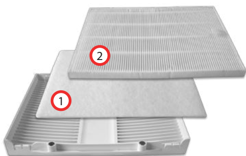
Abb. 6.3.2.2.3: Reinigungsfilter-Set einsetzen
