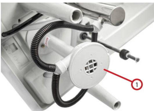
Abb. 6.3.4.6: Pumpenkörper reinigen
