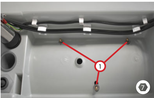
Abb. 7.4.2.5: Verschraubungen lösen
