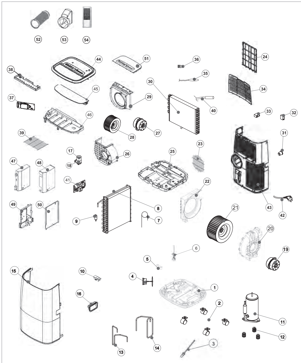
Abb. 14: Gerätedarstellung SKM 250-330 Eco
