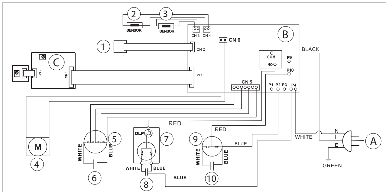
Abb. 12: Elektrisches Anschlussschema
