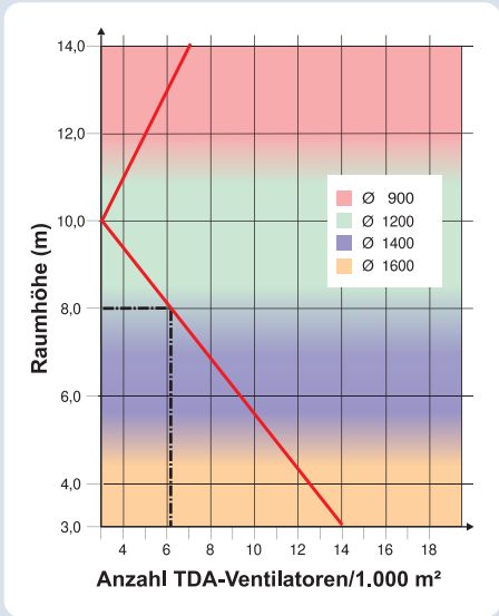
Auswahldiagramm Anzahl Geräte/1.000 m²: In Abhängigkeit von der Raumhöhe (senkrechte Achse) waagerecht nach rechts bis zum Schnittpunkt mit der roten Kennlinie. Von dort senkrecht nach unten. Die waagerechte Achse gibt die Anzahl der benötigten TDA-Ventilatoren pro 1.000 m² an. Die Größe der Ventilatoren ergibt sich aus der Hintergrundfarbe des Schnittpunktes mit der roten Linie.
