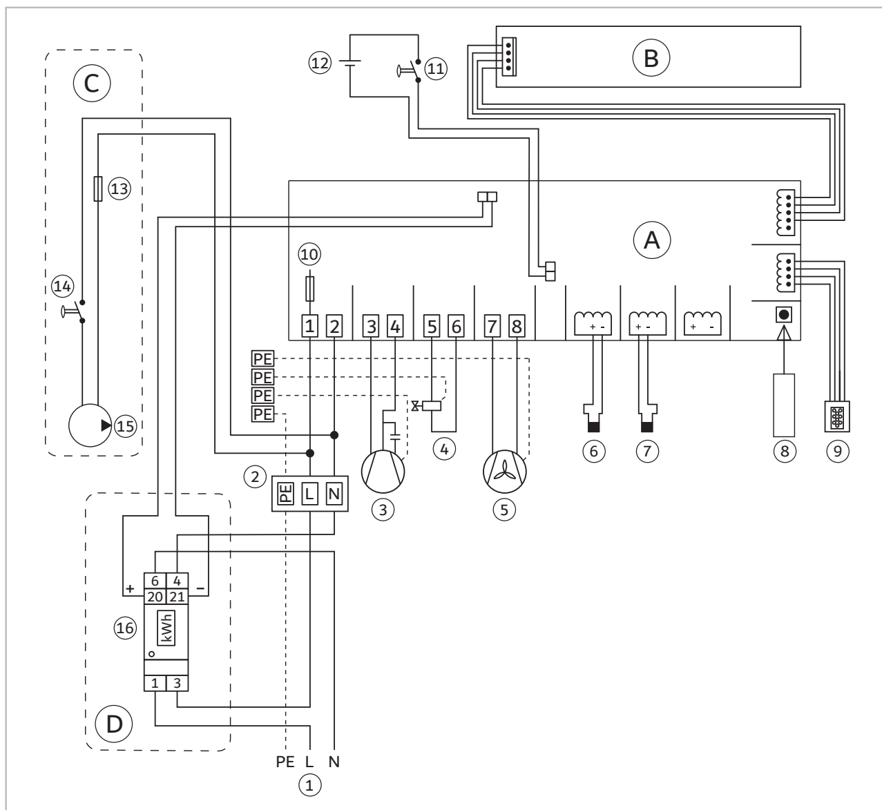
Abb. 7: Elektrisches Anschlussschema
